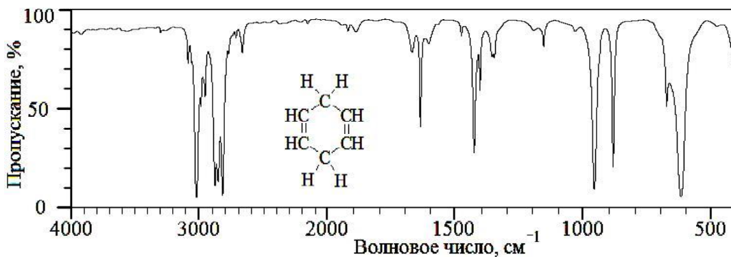
Рис. 3. Циклогекса-1,4-диен:
