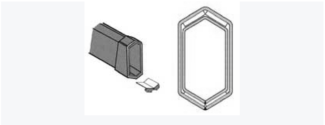
Рис. 2. Шестигранний (гексагональний) профіль стріли кранів-маніпуляторів.
