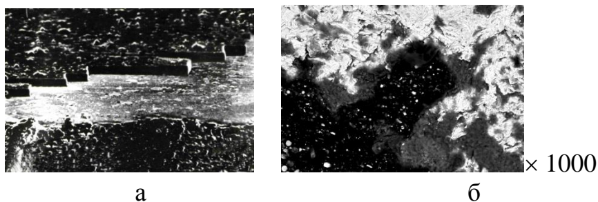
а – відшарування покриття \text{TiN-Cr}_2\text{N} товщиною 8 мкм; б – руйнування покриття \text{TiN-Cr}_2\text{N} товщиною 1 мкм Рисунок 1 – Відшарування покриття \text{TiN-Cr}_2\text{N}
