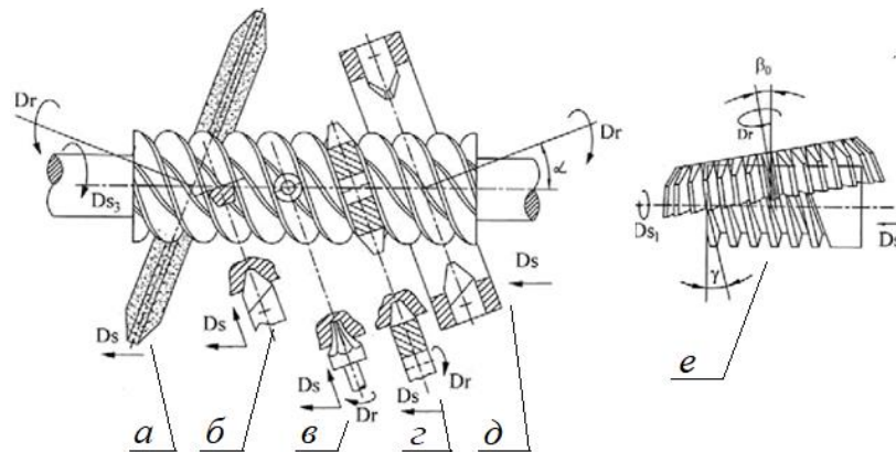
Рис. 3. Схеми методів обробки черв'ячних зуб'ів [4]
