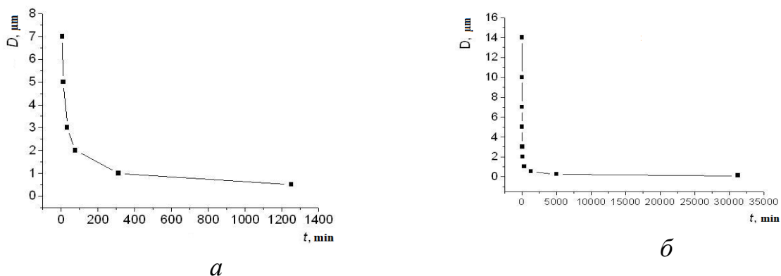
Рис. 1. Залежність мінімального розміру осаджених частинок WO_3 від часу осідання в етиловому спирті при короткочасному (а) та довготривалому (б) осадженні
