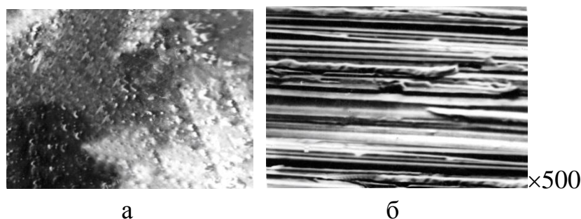
а – з покриттям \text{TiN-Cr}_2\text{N} товщиною 4 мкм; б – після термообробки і шліфування без покриття Рисунок 2 – Поверхня фрагмента ножа зі сталі 65Г
