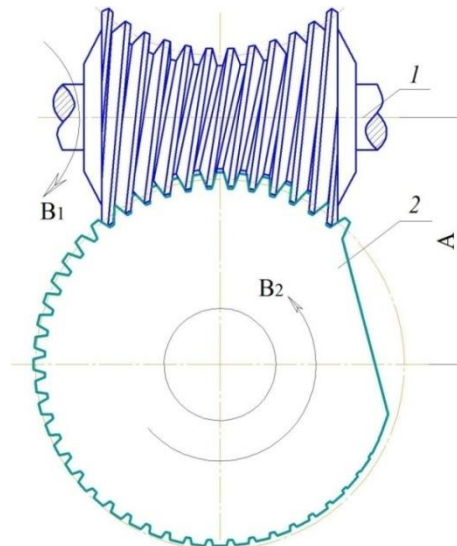
Рис. 5. Схема багаторізевої головки для нарізання глобоїдного черв'яка за методом кругового протягування
