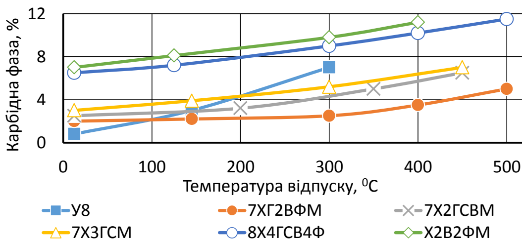
Рисунок 1 – Вміст карбідів в сталях в залежності від температури відпуску
