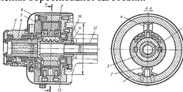
Рис. 2. Лопатевий гідропривід
