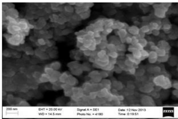
Рис. 2. Електронно-мікроскопічне зображення осаджених частинок оксиду WO_3 після 24 год. (100000×)
