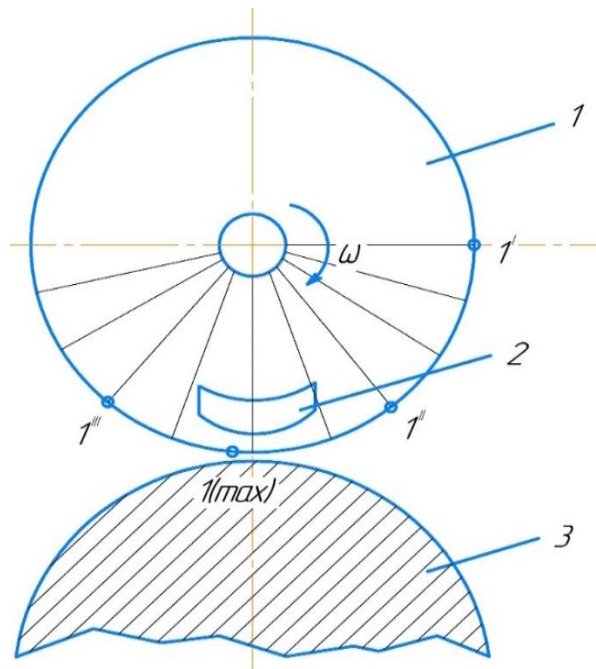
Рисунок 1 – Схема установки
